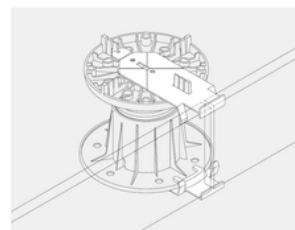
Beslag för montering av kantlist.
